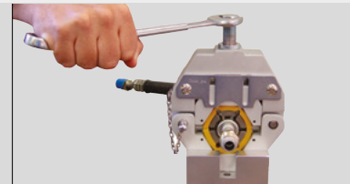
Feche o garfo, insira o pino e gire o parafuso do cabeçote
