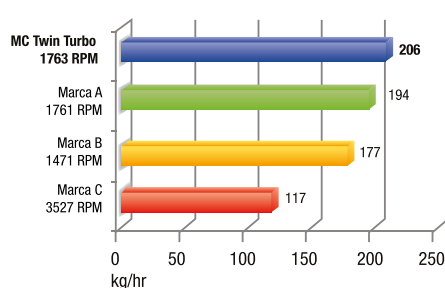
Recuperação de Líquido (In) kg/hora Temperatura: 79 a 82°F / Gás Refrigerante: R22
