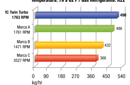
Push-Pull (In) kg/hora Temperatura: 79 a 82°F / Gás Refrigerante: R22
