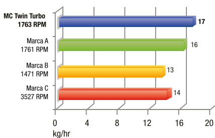
Recuperação de Vapor (In) kg/hora Temperatura: 79 a 82°F / Gás Refrigerante: R22
