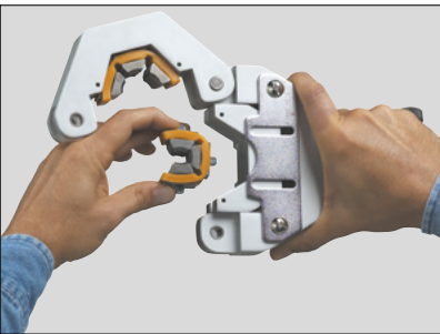
O molde prende-se rapidamente ao encaixe da prensa, sem a necessidade de pinos e parafusos
